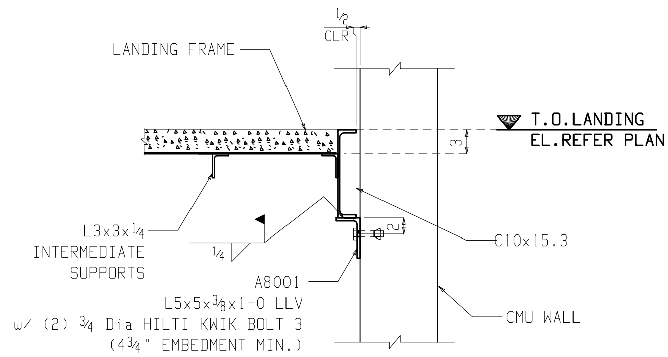
B DETAIL-B E8004
