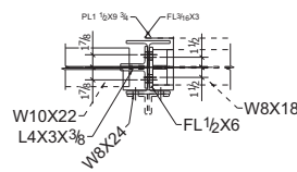
I - J E5
