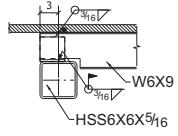
B - B E2 Ref-section. 4/S-121
