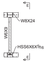
DETAIL 2 E2
