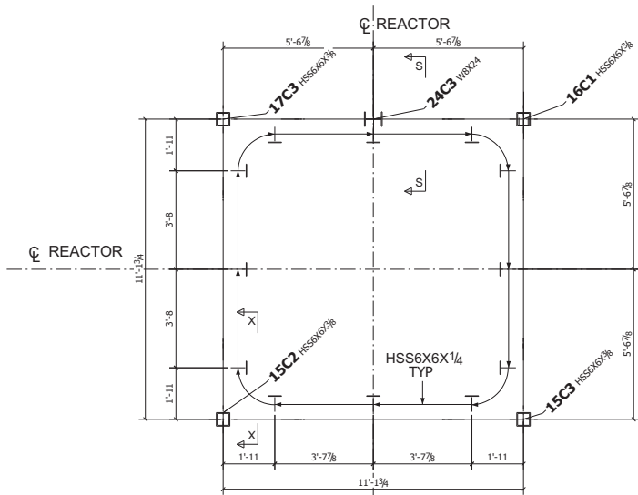
DETAIL 1 E2
